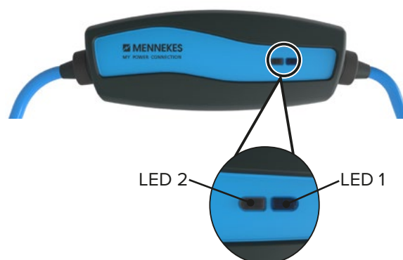
Obr.: Rozmístění kontrolky na horní straně skříně
