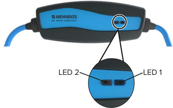
Resim: Mahfazanın üst tarafındaki LED'lerin yerleşim düzeni
