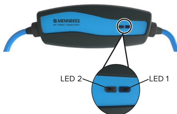
Εικόνα: Διάταξη των λυχνιών LED στην επάνω πλευρά του περιβλήματος
